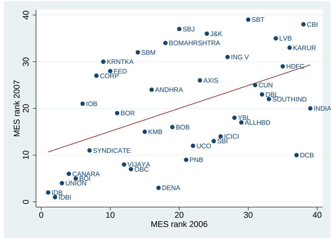
Figure C6. : MES Rank for Jan '07–Dec '07 versus MES Rank for Jan '06–Dec '06
